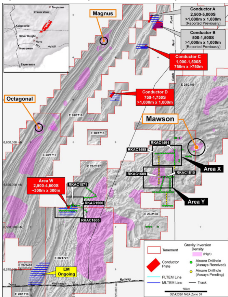
Fig.6. Area W – Anomalous geochem (Ni-Cu) and EM target to test
